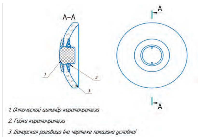
Рис. 3. Схема расположения конструкции кератопротеза с фиксированной роговицей донора.
